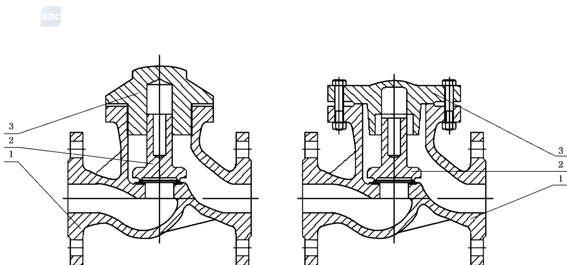
图 3 内螺纹连接升降式止回阀
