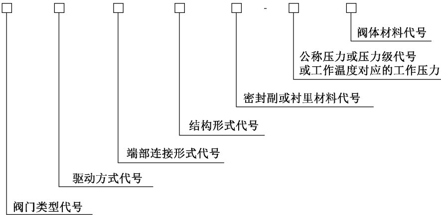
图 1 阀门型号
